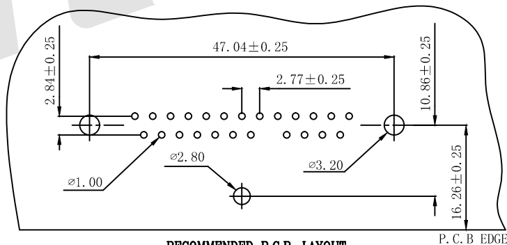
RECOMMENDED P.C.B. LAYOUT INSPECTION DIMENSION:(A)~(D)
